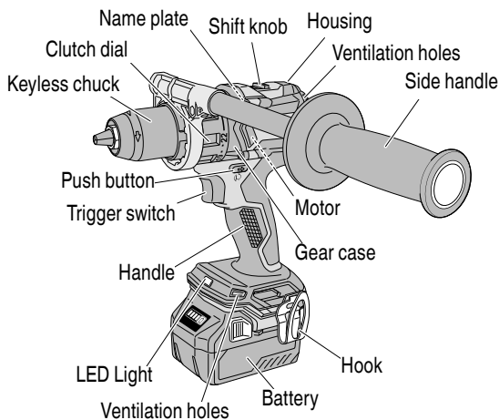
<DS18DC / DV18DC / DV36DC> Fig. 3
