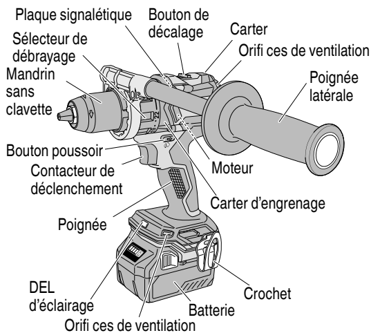
<DS18DC / DV18DC / DV36DC> Fig. 3
