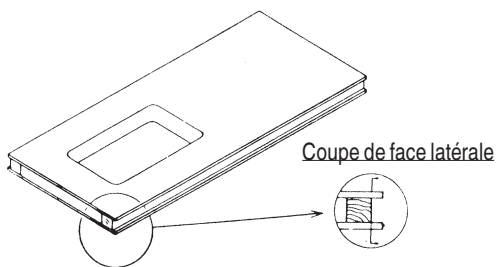
Fig. 2-E (Rabotage latéral d'une porte à ras)
