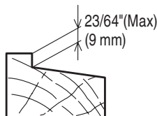
Fig. 2-D (Taillage en pointe)
