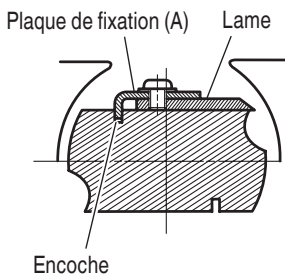
Fig. 10 (Installation correcte)
