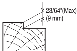
Fig. 2-C (Feuilleure)
