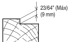
Fig. 2-C (Ranurado)
