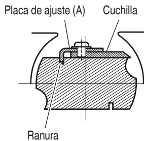
Fig. 10 (Instalación correcta)
